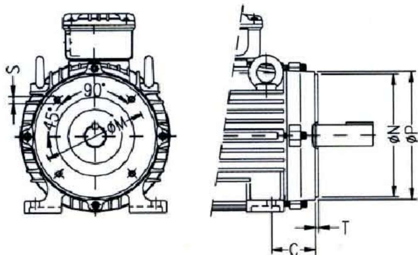
Стандартное исполнение / Standard Frame / Standard-Baugröße
