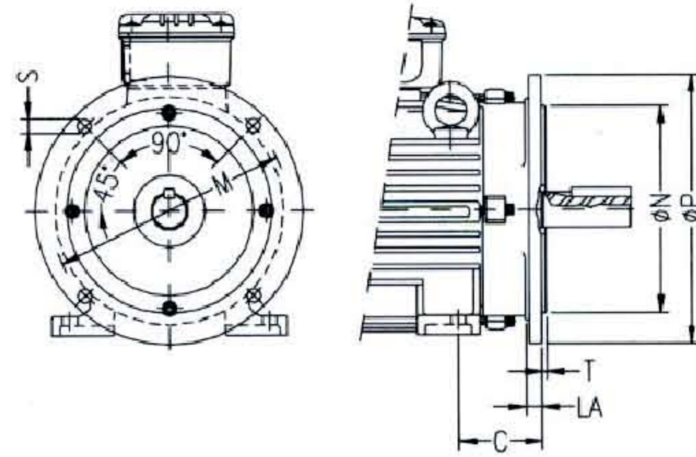
Стандартное исполнение / Standard Frame / Standard-Baugröße
