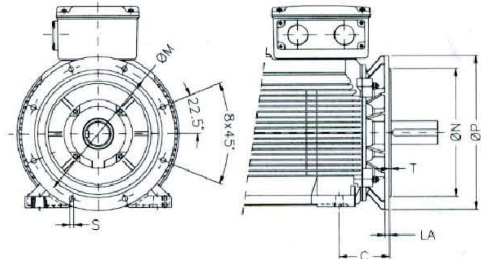
Станина 315B / 315B Frame / Baugröße 315B
